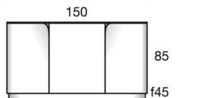
910A151Z MOD. SIDEBORD 3 DOORS APARADOR 3 PUERTAS Top Tapa: Chapa / L.Marmol Venner / L. marble Walnut / Ash Nogal / Fresno: 1657 pts Lacquered Lacado: 1574 pts Customer veneer Ch. cliente: 1773 pts
