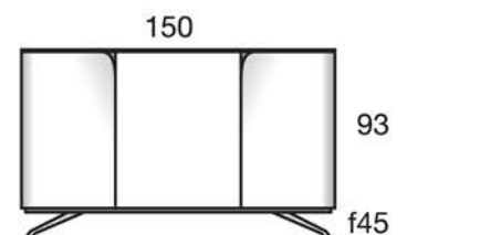
910A151P MOD. SIDEBORD 3 DOORS APARADOR 3 PUERTAS Top Tapa: Chapa / L.Marmol Verner / L. marble Walnut / Ash Nogal / Fresno: 1687 pts Lacquered Lacado: 1603 pts Customer veneer Ch. cliente: 1805 pts
